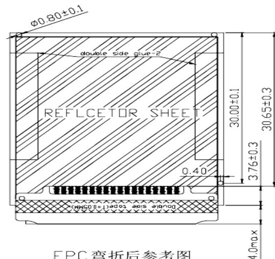
FPC 弯折后参考图
